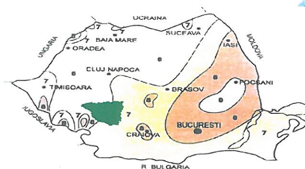
HARTA CU ZONELE DE RISC SEISMIC
